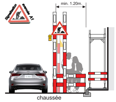
E 3 Fermeture du trottoir (déviation des piétons sur la chaussée)
