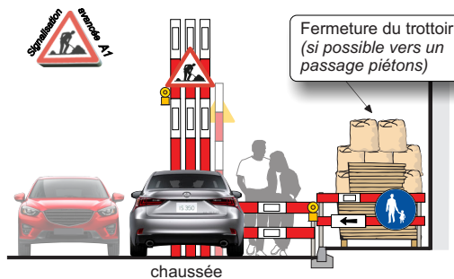
I 5 Installation sur chaussée & place de parc (avec déviation des piétons sur trottoir adjacent)
