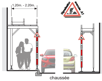
E 2 Normal & tunnel (en bordure ou sur chaussée)
