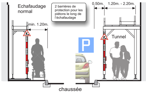
E 1 Normal & tunnel (sur trottoir, sans perturbation pour les piétons)
