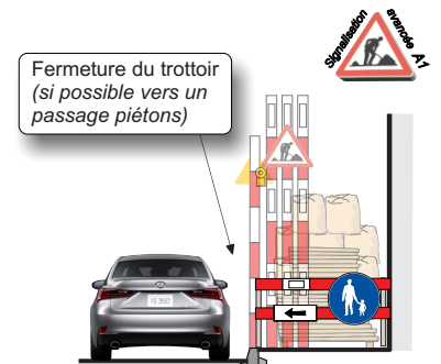
I 3 Installation sur trottoir (déviation des piétons sur trottoir adjacent)
