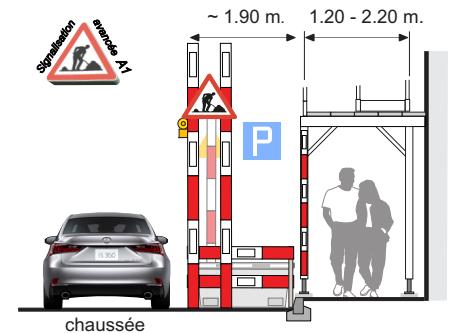
E 6 Tunnel (avec benne sur place de parc)
